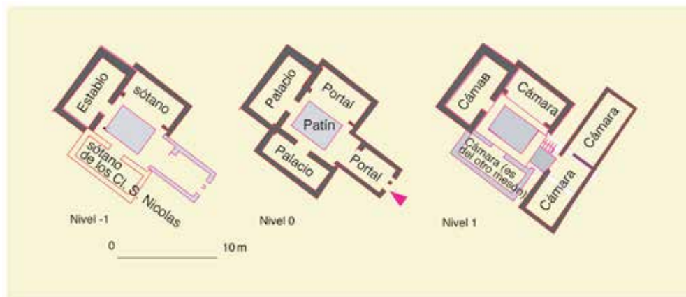
Calle de las Armas, nº 3: restitución y planimetría de la casa AA-3 en el año 1492 (la casa fue derribada en la primera mitad del siglo XX).
