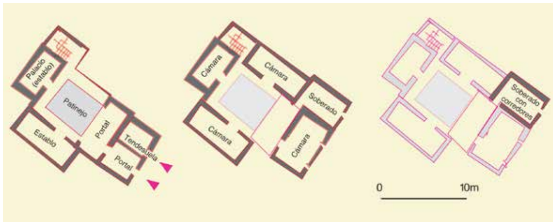
Calle de las Armas, n° 1: restitución y planimetría en el año 1492 de la casa AA-3, derribada en la primera mitad del siglo XX.
