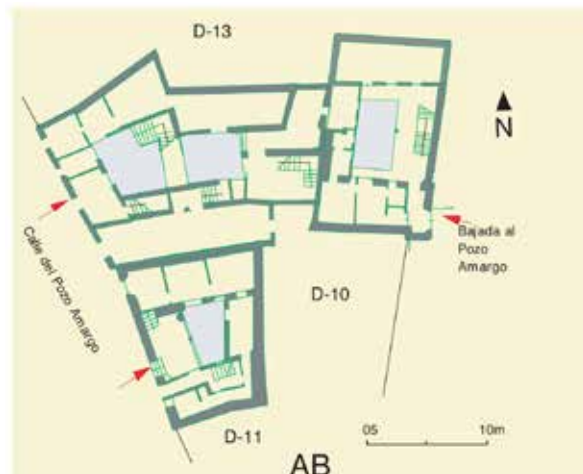
A, Bajada del Pozo Amargo, nº 12; calle del Pozo Amargo, nºs 7 y 9: plano actual B, Calle del Pozo Amargo, nº 9: plano actual; restitución y planimetría de la casa D-12c
