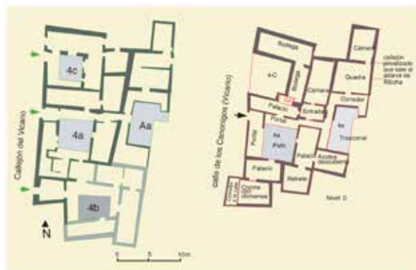
Fig. Callejón del Vicario nos 7, 9, 11: plano actual
