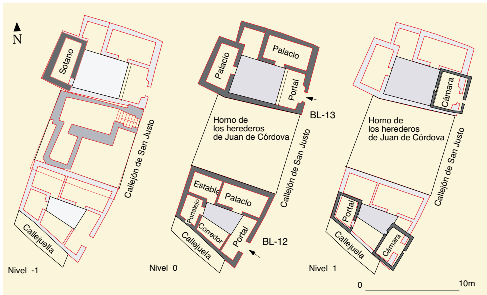
Callejón de San Justo, nºs 6, 8, 10: restitución y planimetría de las casas BL-12 y BL-13 en el año 1492.
