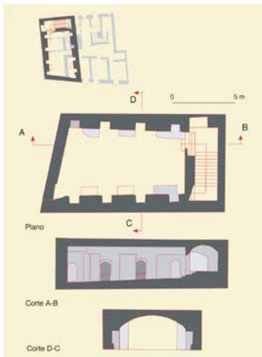
Fig. 252. Calle Sixto Ramón Parro, n° 1: estado actual del sótano construido en el año 1560 en la bodega de los frailes.
