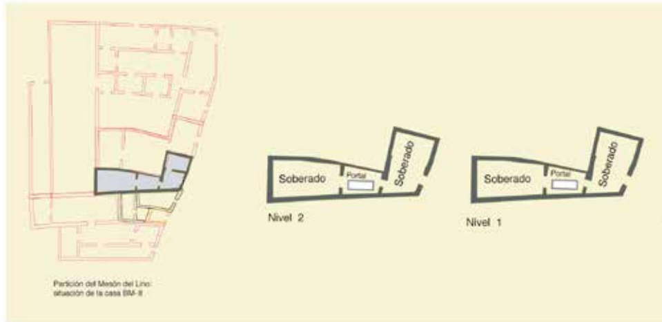
Calle de Santa Justa, nº 3: restitución y planimetría de la casa BM-8.
