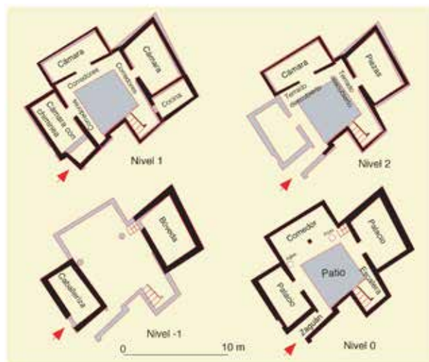
Callejón de Córdoba, nº 5: restitución y planimetría de la casa en el año 1520
