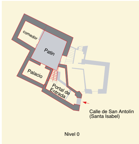
Fig. 313. Calle de Santa Isabel, nº 18: restitución y planimetría de la casa F-4b.
