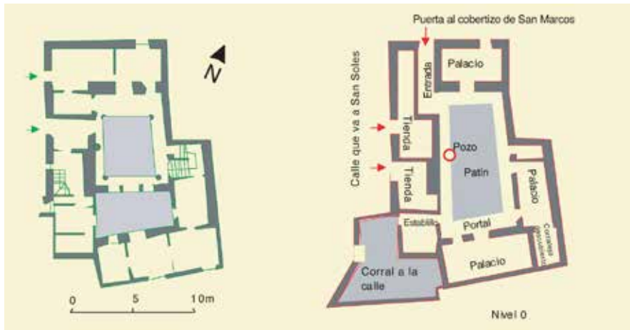
Calle de Santa Úrsula, n° 11: plano actual; restitución y planimetría de la casa AQ-6.
