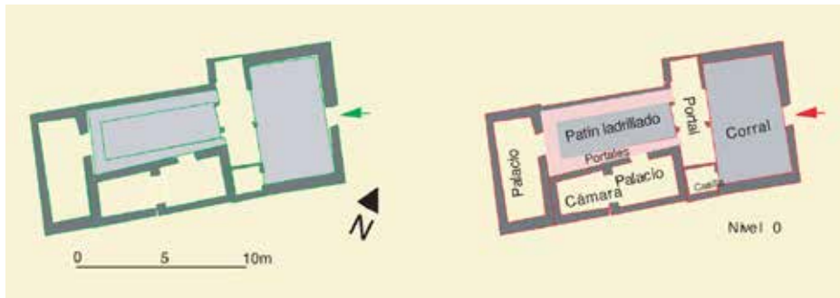
Travesía de Santa Isabel, n° 4: plano restituído; restitución y planimetría de la casa AQ-7
