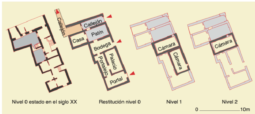
Calle de San Miguel, n°14, 16: restitución y planimetría de la casa AOO-11 en 1492.
